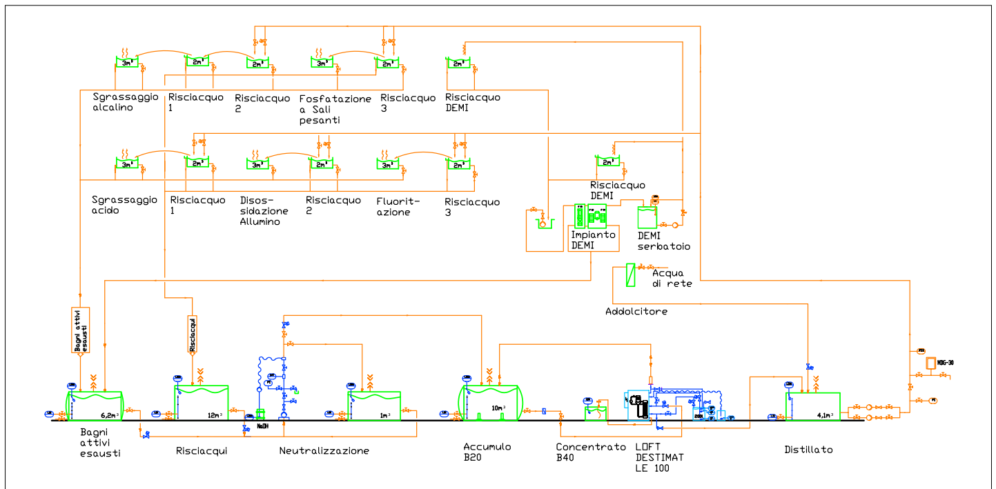
Fig. 9 - Il layout dell'impianto di trattamento delle acque: in blu sono indicate le componenti fornite e installate da Loft; in verde sono indicati gli impianti di pretrattamento, il demineralizzatore e i serbatoi di accumulo e stoccaggio reflui, distillato e concentrato
